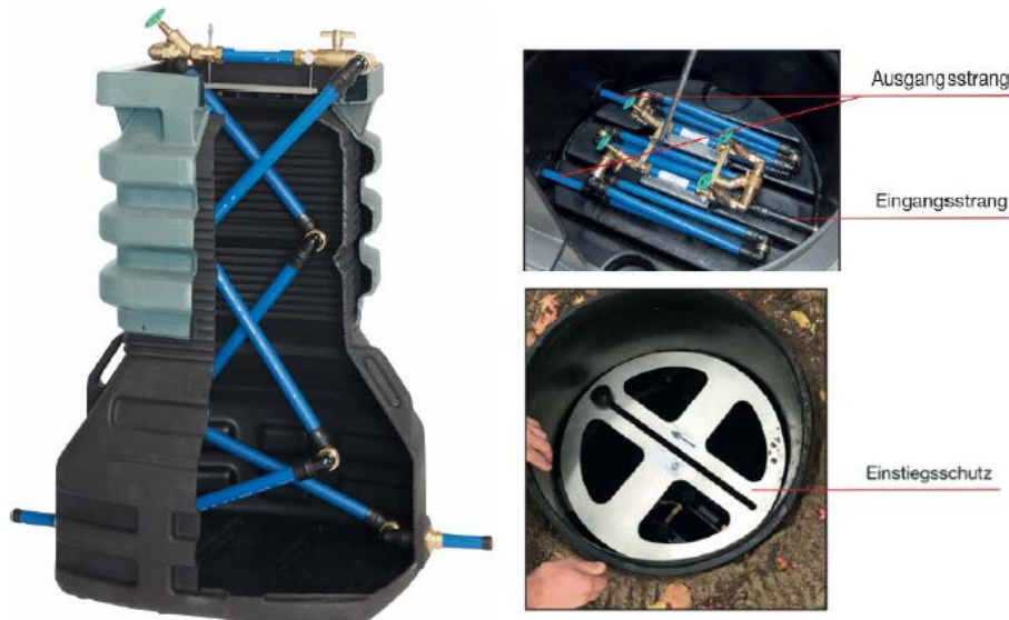
Abb. 2: Beispiel ausziehbarer bzw. nicht begehbaren Wasserzählerschacht
